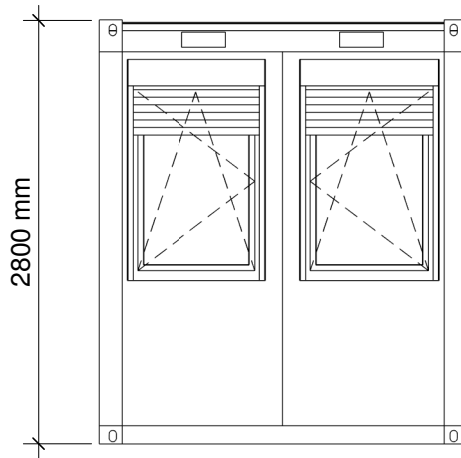
Ansicht Ost
