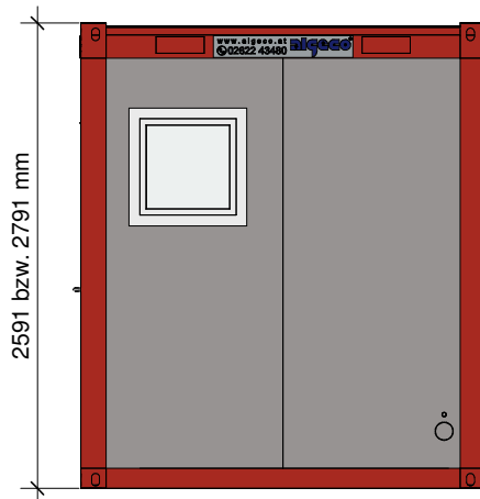
Ansicht Ost
