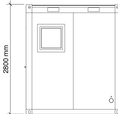
Ansicht Ost
