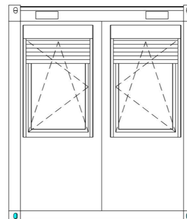
Pogled Vzhod
