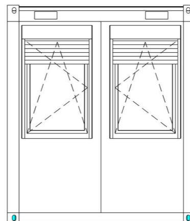
Pogled Vzhod
